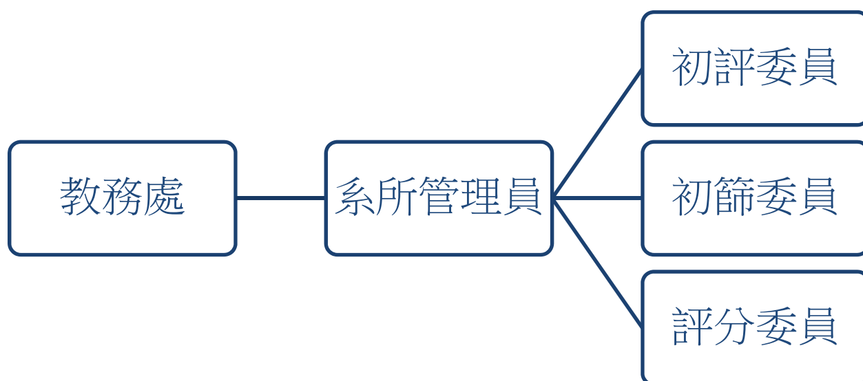
圖 1 帳號關係圖
